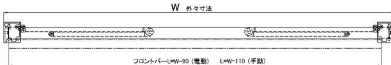
平面図
