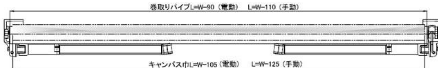
正面図
